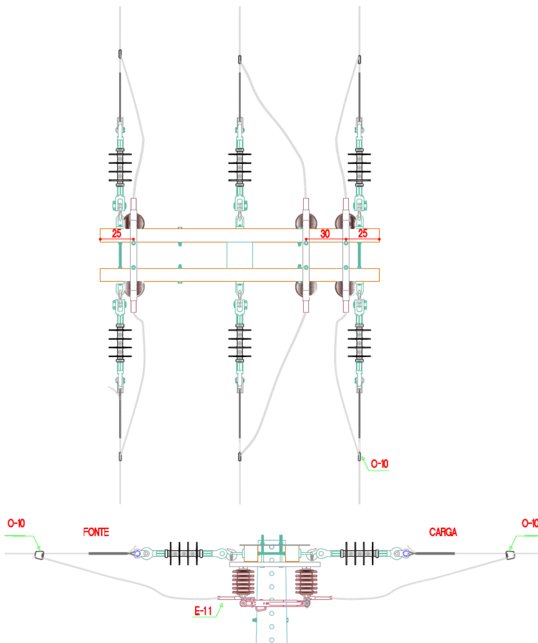
Figura 8 – Estrutura N4 com Seccionador Unipolar em Primeiro Nível Dimensões em cm
