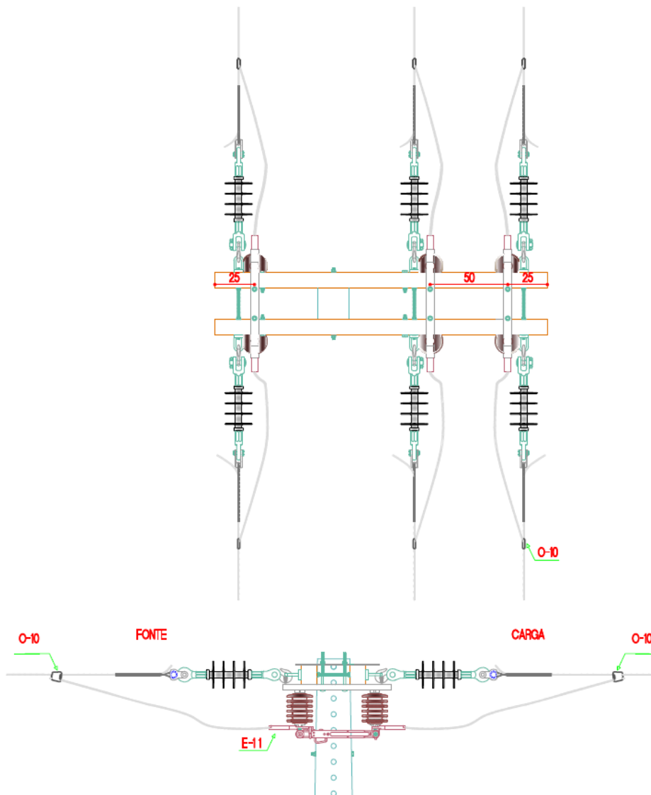
Figura 6 – Estrutura M4 com Seccionador Unipolar em Primeiro Nível Dimensões em cm
