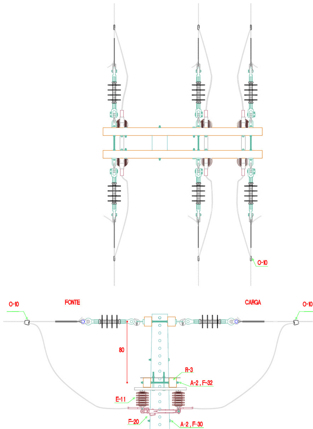
Figura 9 – Estrutura M4 com Seccionador Unipolar em Segundo Nível Dimensões em cm
