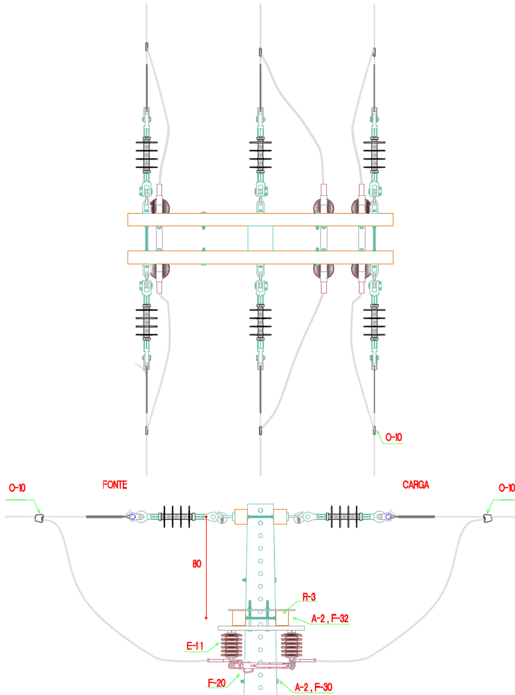
Figura 11 – Estrutura N4 com Seccionador Unipolar em Segundo Nível Dimensões em cm
