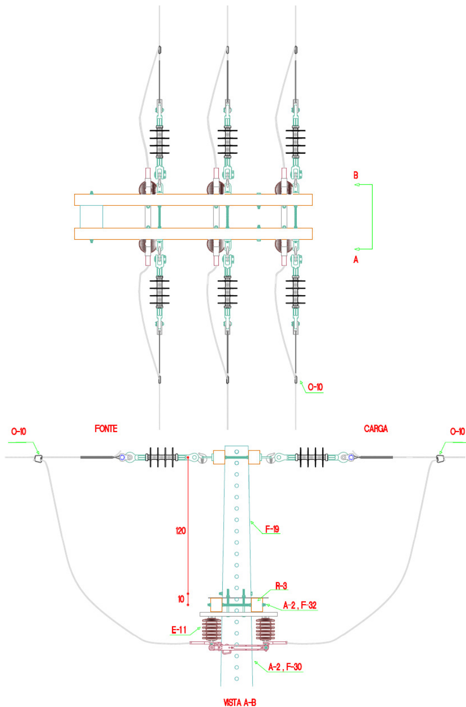
Figura 10 – Estrutura B4 com Seccionador Unipolar em Segundo Nível Dimensões em cm
