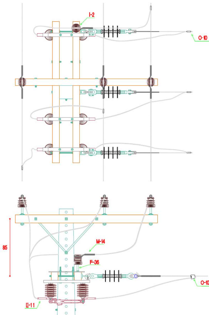
Figura 1 – Estrutura M1-N3 com Seccionador Unipolar Dimensões em cm
