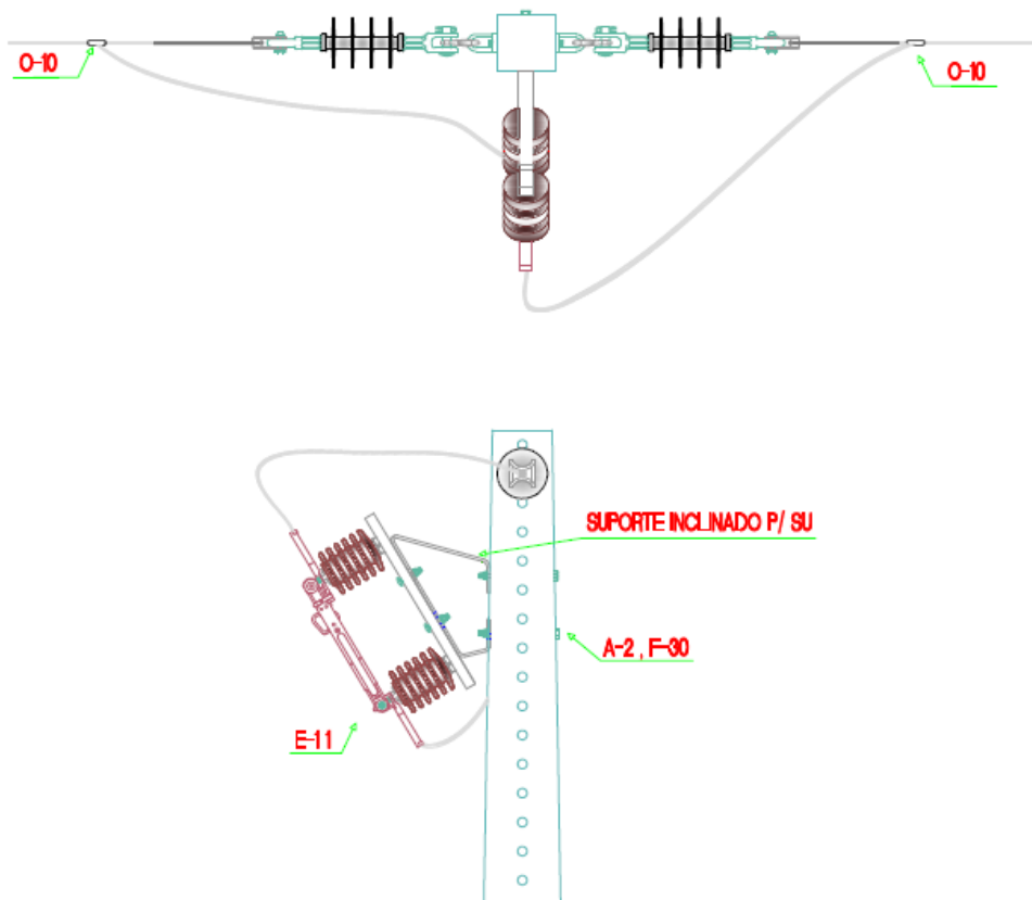
Figura 12 – Estrutura U4 com Seccionador Unipolar Dimensões em cm
