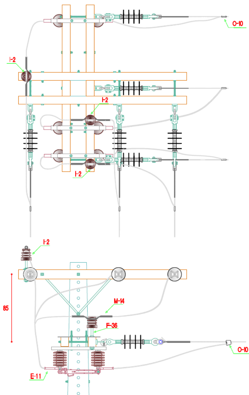
Figura 2 – Estrutura M3-N3 com Seccionador Unipolar Dimensões em cm
