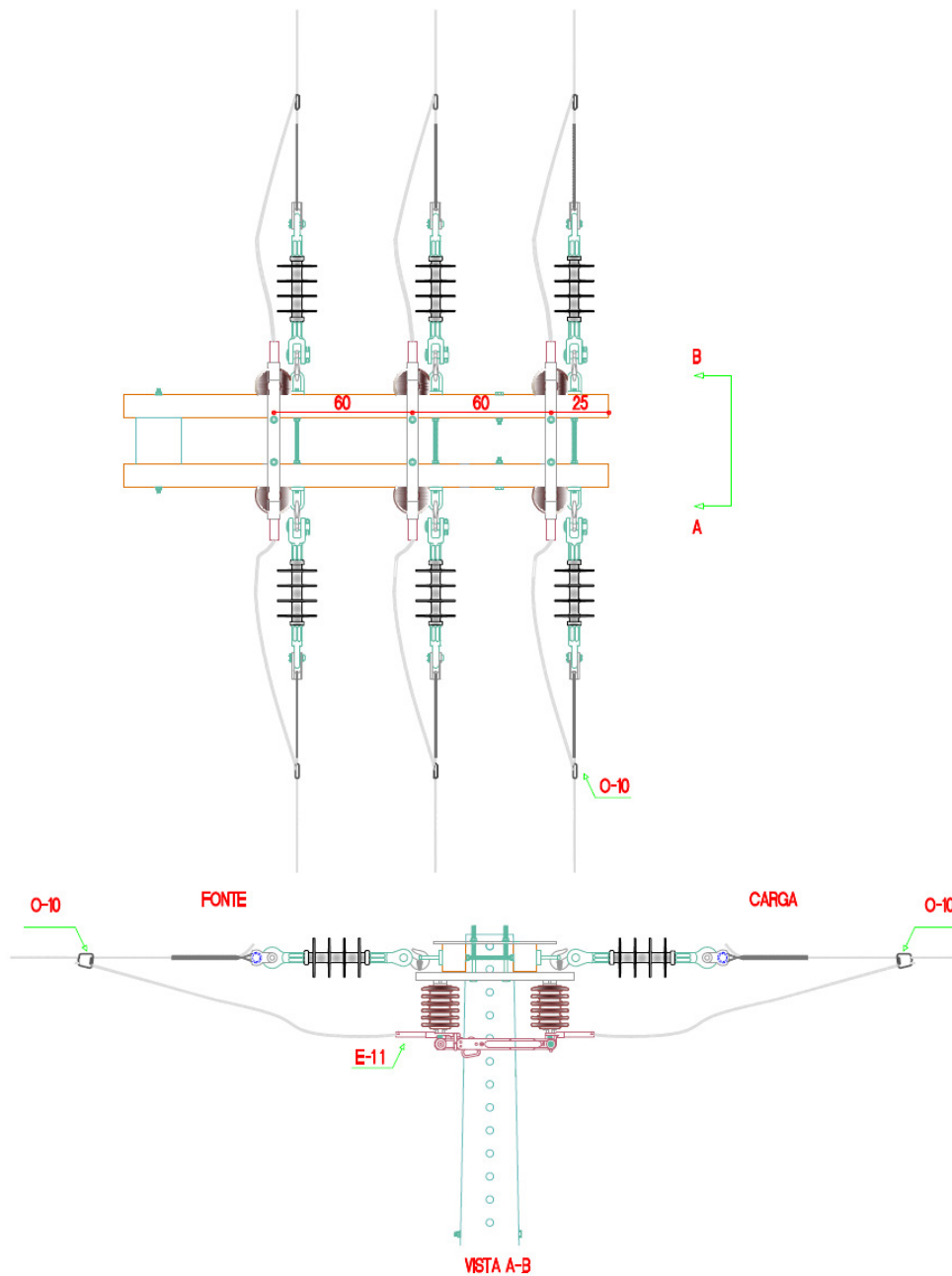
Figura 7 – Estrutura B4 com Seccionador Unipolar em Primeiro Nível Dimensões em cm
