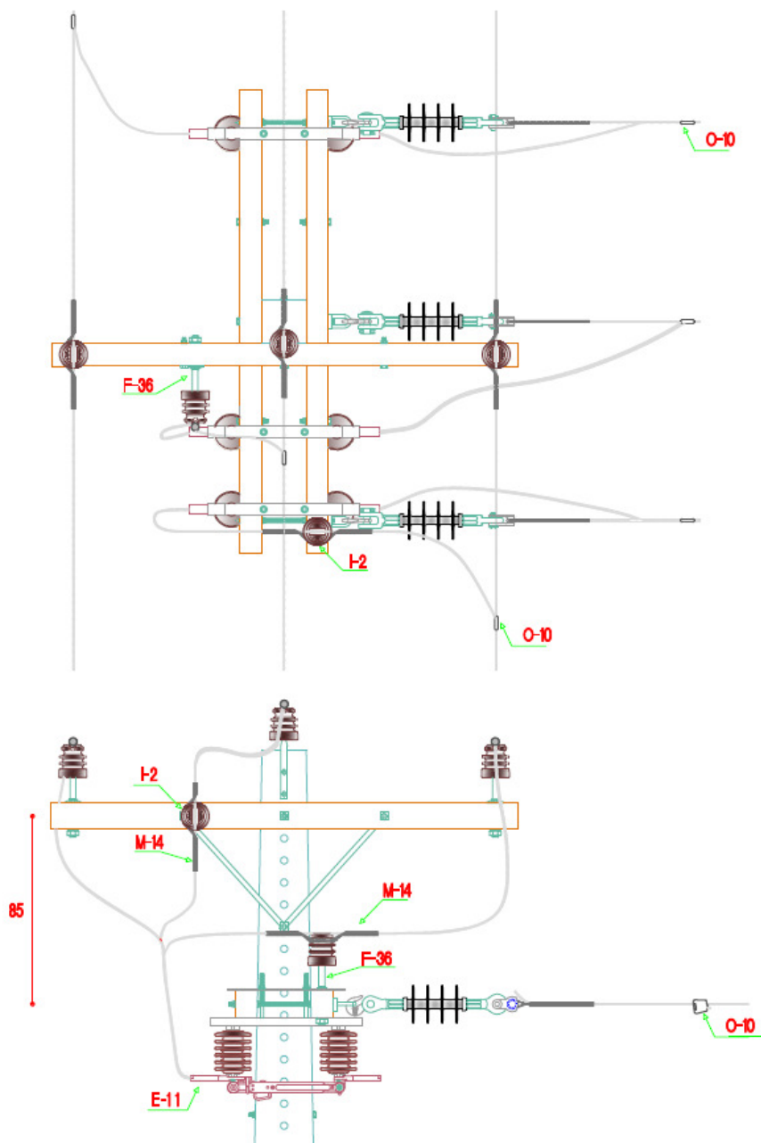
Figura 5 – Estrutura T1-N3 com Seccionador Unipolar Dimensões em cm
