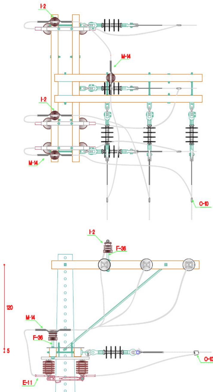
Figura 4 – Estrutura B3-N3 com Seccionador Unipolar Dimensões em cm
