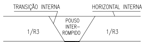
CORTE B-B
