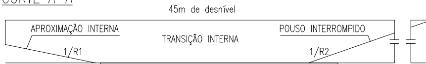
CORTE A-A
