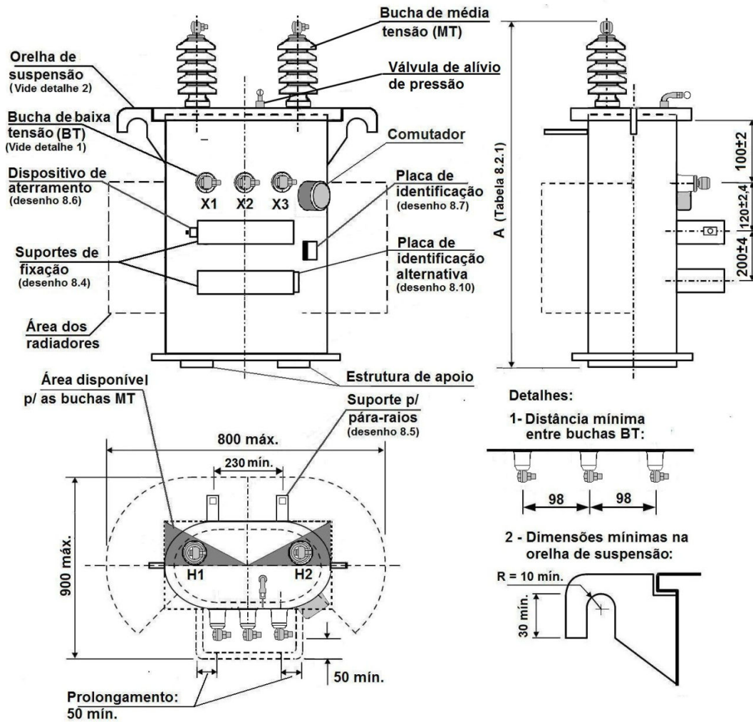
Figura 8.2.1 – Dimensões e Disposição dos Componentes
