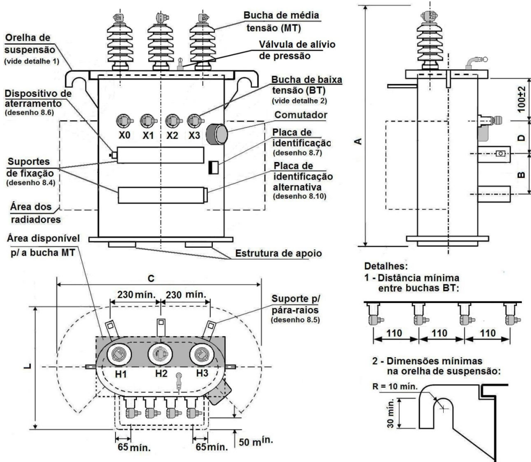
Figura 8.3.1 – Disposição e Dimensões dos Componentes
