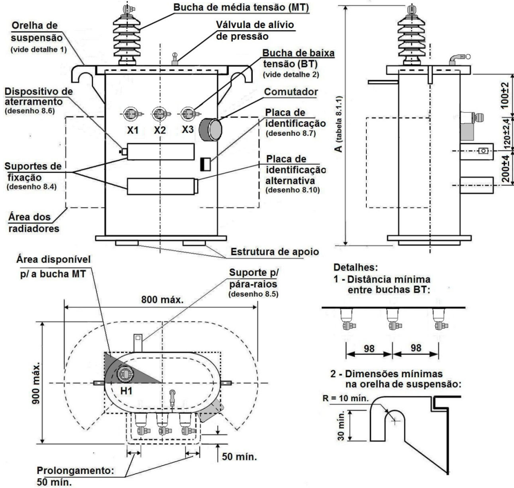
Figura 8.1.1 – Dimensões e Disposição dos Componentes
