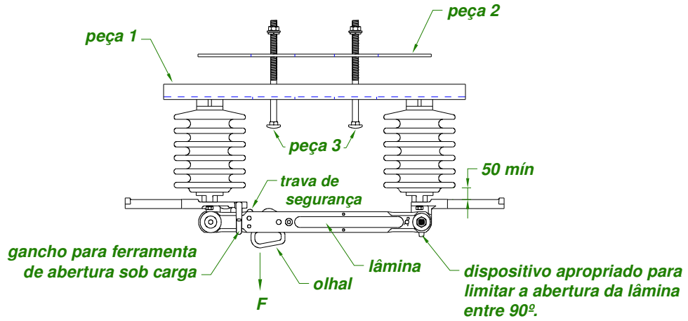
Detalhe 1 terminal tipo nema
