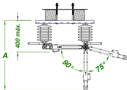
Detalhe 2 fixação em cruzetas
