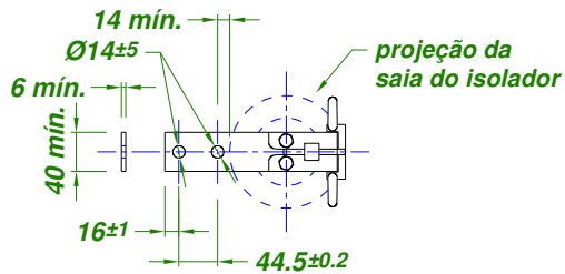
Detalhe 1 terminal tipo nema
