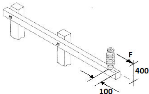
Figura 8.2 – Ensaio de Tração Longitudinal
